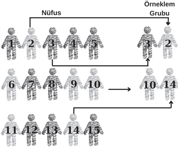
Şekil 5.1 Basit Rassel Örnekleme
